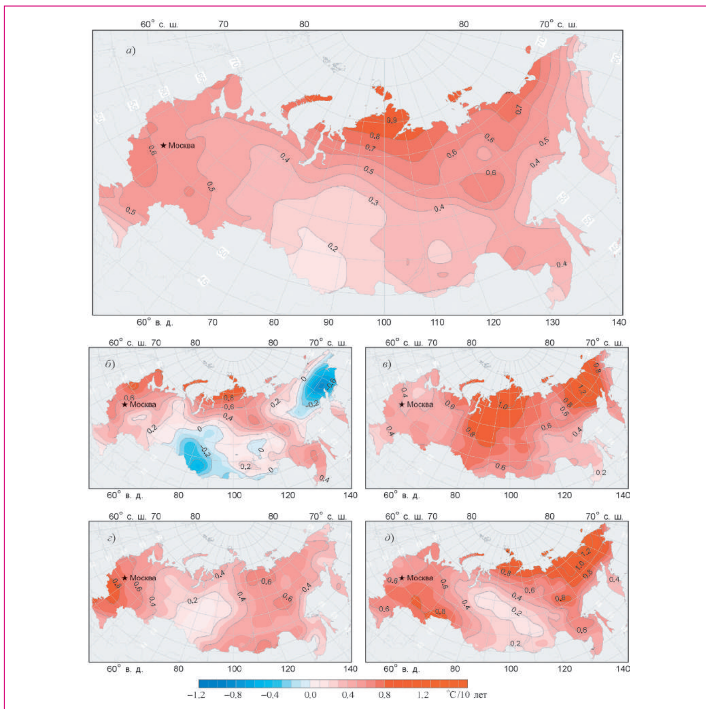
Рис. OP1.3. Географическое распределение коэффициентов линейного тренда среднегодовой (а) и средней сезонной температуры (б–д) на территории России за 1976–2012 гг.: б) зима; в) лето; г) весна; д) осень. Оценки получены по данным наблюдений на сети Росгидромета (данные накоплены за период с 1886 г.; база данных под-держивается ИГКЭ).
