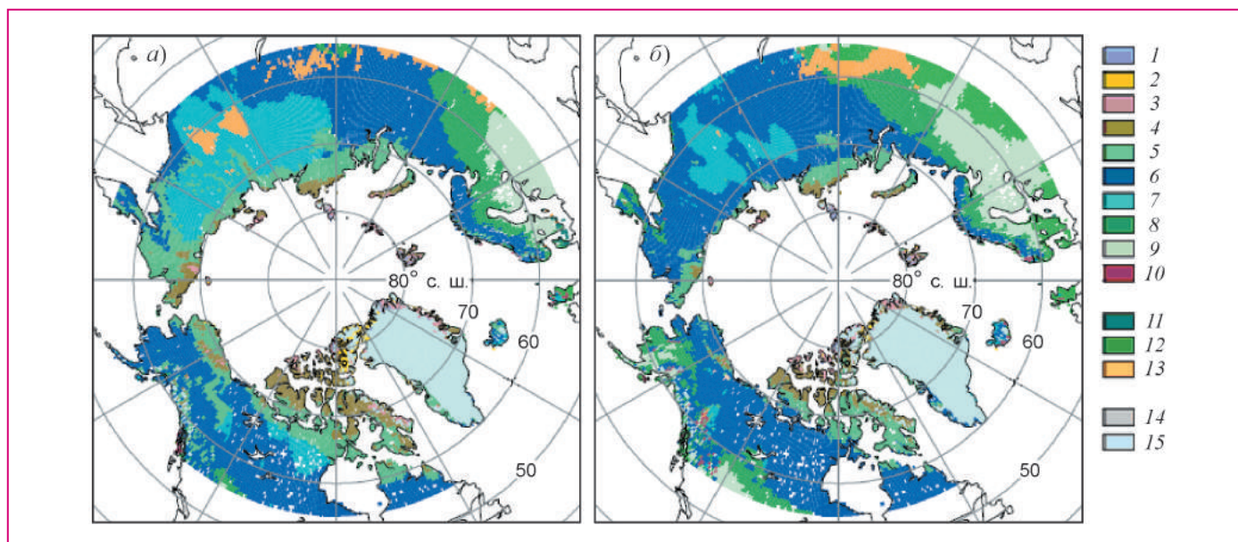
Рис. ОР4.5. Распределение растительности севернее 55° с. ш.: а) современное, согласно базе данных SAVM/GLC2000; б) рассчитанное по модели BIOME4 при глобальном потеплении на 2°С. 1) бесплодные земли; 2) граминоидная тундра; 3) тундра со стелящимися карликовыми кустарниками; 4) тундра с прямостоящими карликовыми кустарниками; 5) кустарниковая тундра; 6) вечнозеленая бореальная тайга; 7) листопадная тайга; 8) вечнозеленая средняя тайга; 9) смешанный бореальный лес; 10) смешанный лиственный лес; 11) вечнозеленый лиственный лес; 12) листопадный широколиственный лес; 13) травы и ксерофильные кустарники; 14) голая земля; 15) лед; из (Bala, Caldeira, Mirin, et al., 2005).
